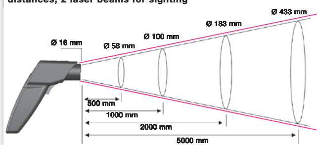
testo 830-T2
